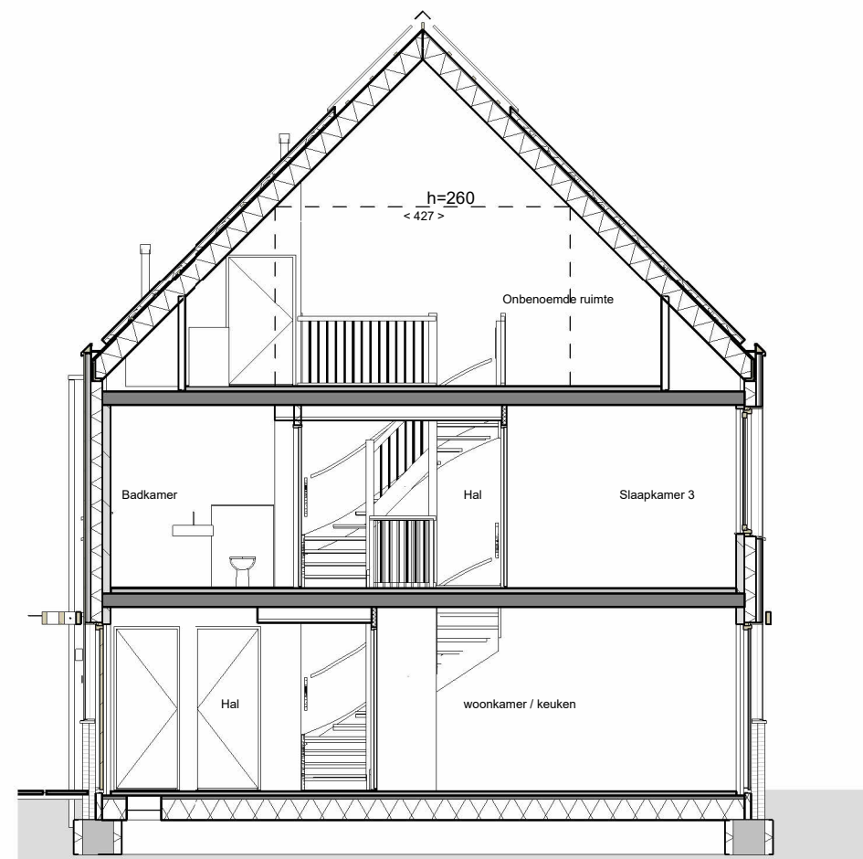
doorsnede
