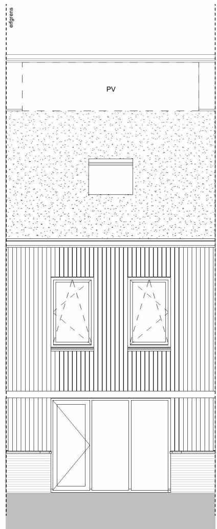
achtergevel
